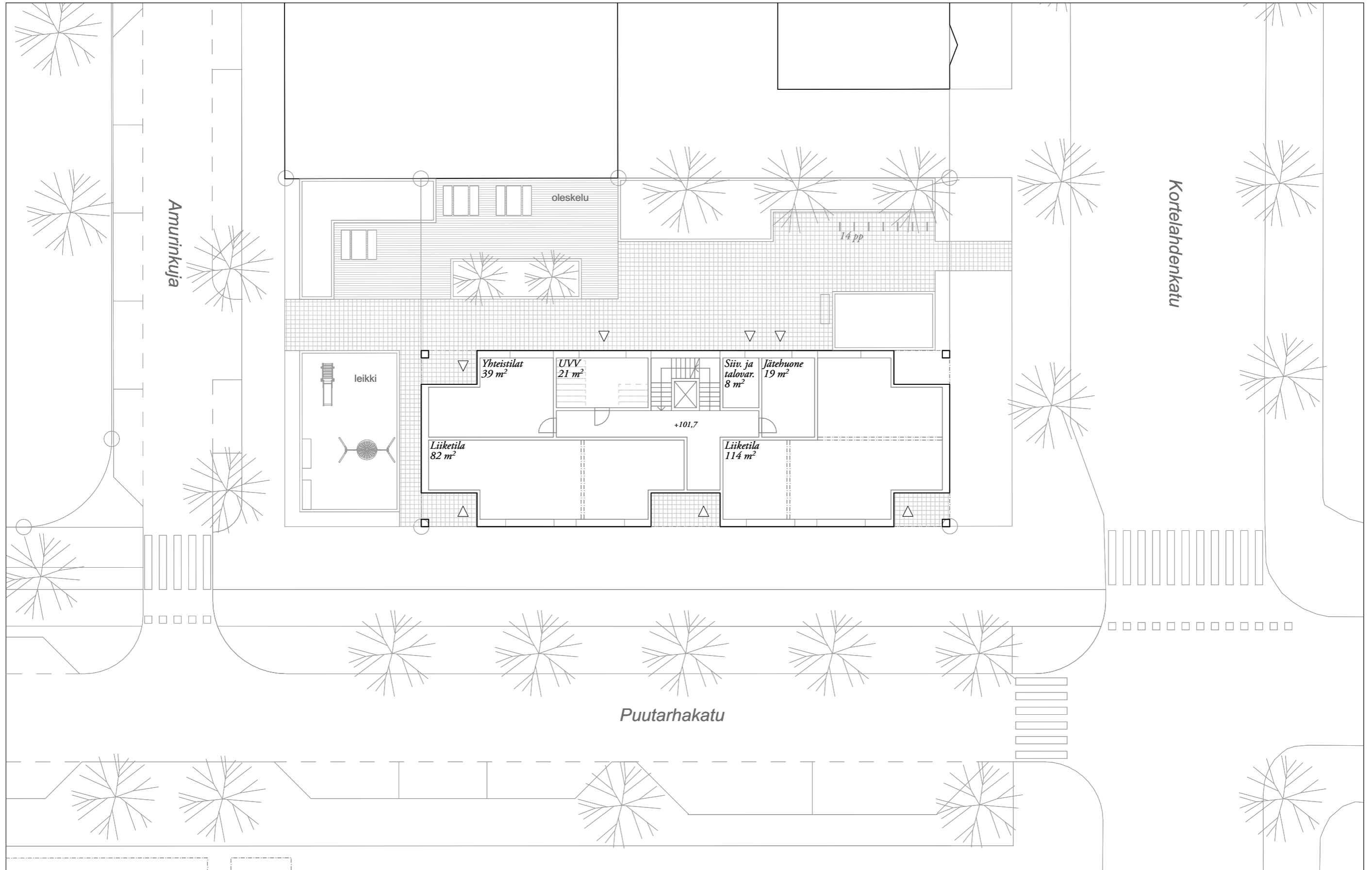
1. kerros 1:250
